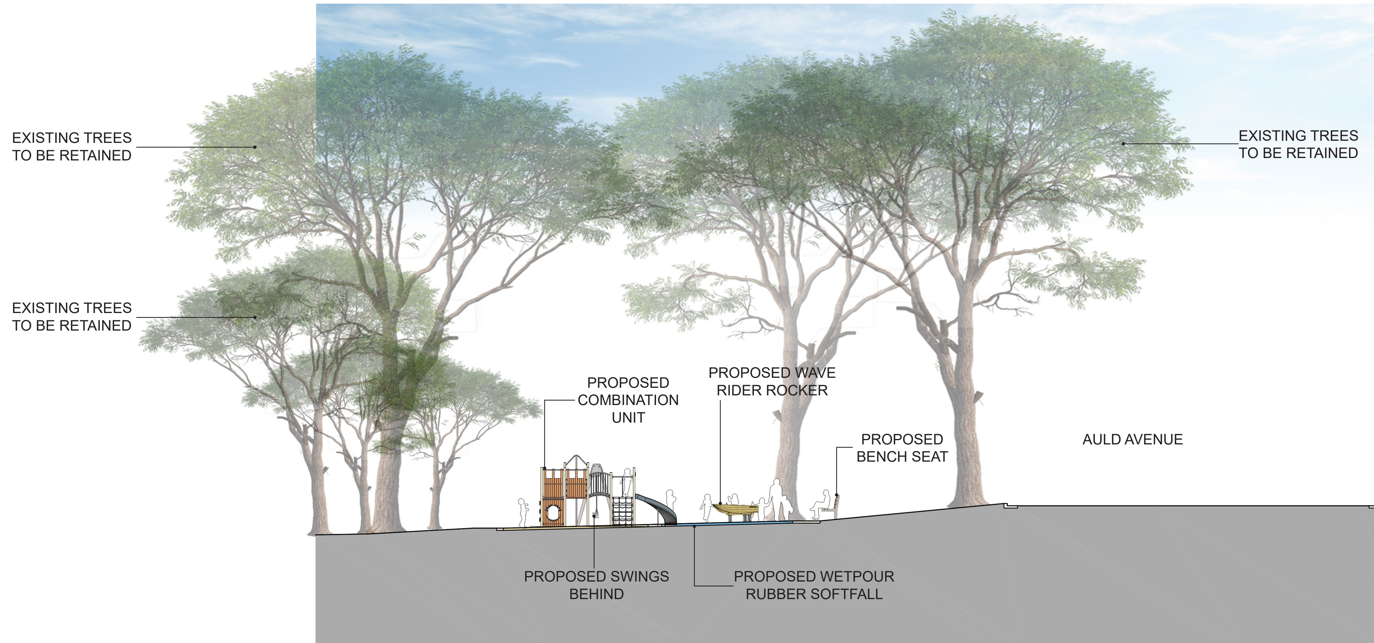
SECTION A-A
